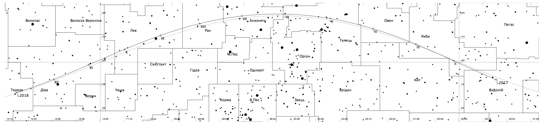
Рис. 7. Видимий шлях Марса
