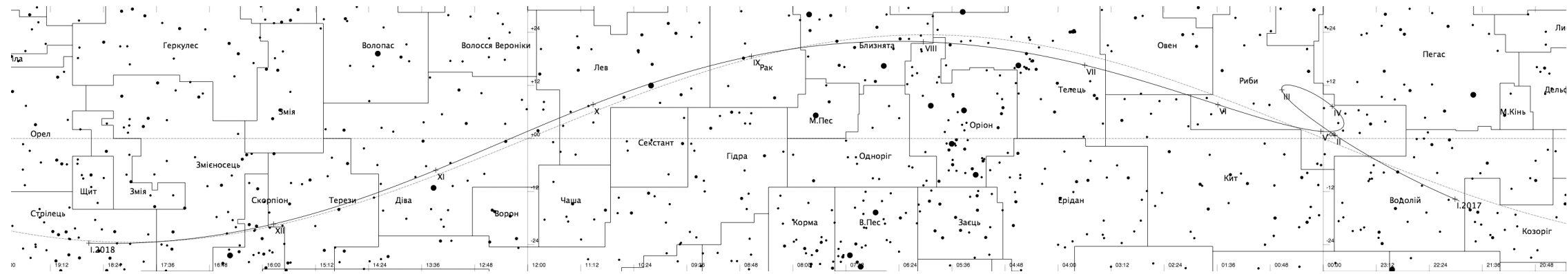
Рис. 6. Видимий шлях Венери
